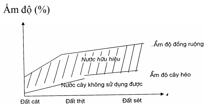
Đồ thị 4.2: Quan hệ giữa độ ẩm đồng ruộng, độ ẩm cây héo, lượng nước hữu hiệu với thành phần cơ giới đất (Theo Brandy, 1984)
