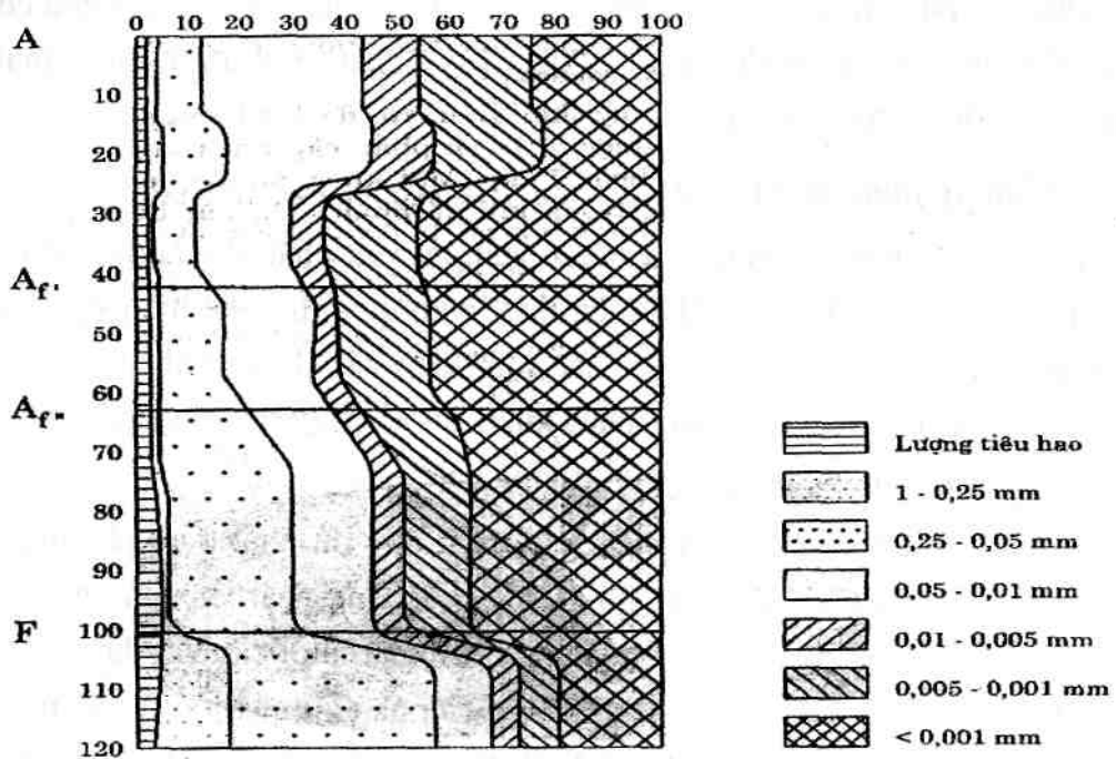
Hình 1.6: Thành phần cơ giới đất feralít nâu đỏ phát triển trên bazan (ferrasols), Nông trường Tây Hiếu, Nghệ An biểu diễn theo phương pháp phẫu diện
