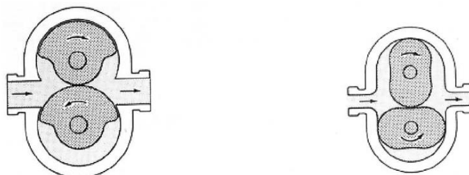
Hình 4.14. Bơm vòng 1 lobe (trái) và nhiều lobe (phải)
