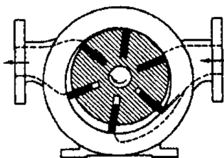
Hình 4.12. Bơm cánh gạt 6 cánh
