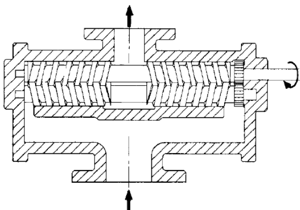
Hình 4.7. Bơm rô to 2 trục vít 2 đầu hút.
