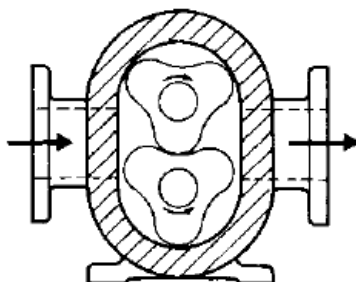
Hình 4.13. Nguyên lý làm việc của một bơm vòng 3 lobe.
