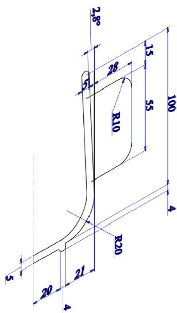
Biên dạng thân ly
