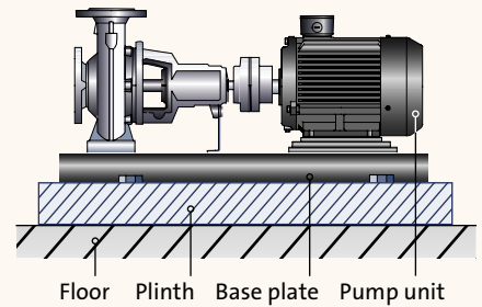
Fig. 2.1.7: Plinth
