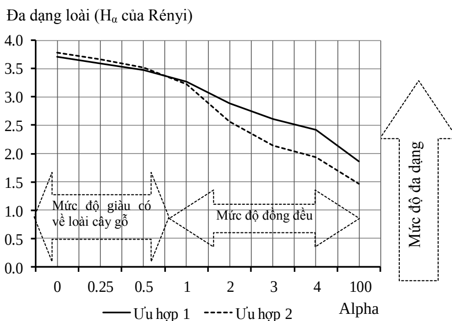
Hình 8.2. Đồ thị biểu diễn hồ sơ đa dạng loài cây gỗ của Rényi đối với hai ưu hợp Dầu rái.
