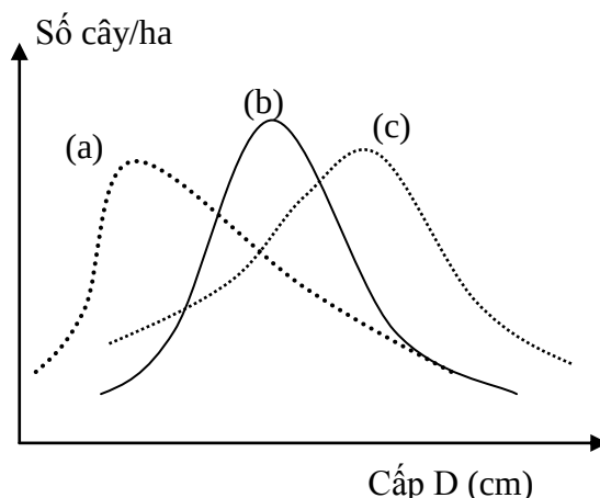
Hình 7.8. Phân bố N/D và N/H trong rừng đồng tuổi.
