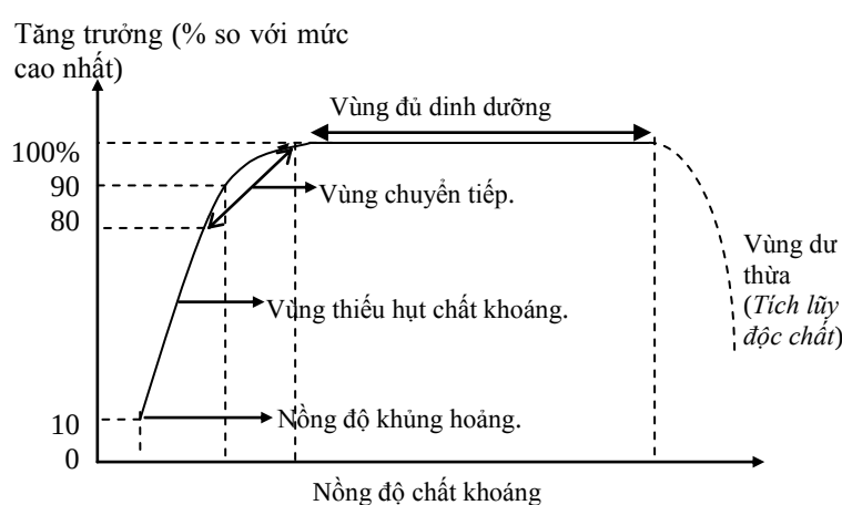
Hình 5.1. Mối quan hệ giữa tăng trưởng của thực vật và nồng độ chất khoáng trong mô của nó (Ulrich và Hill, 1967; Dẫn theo Kimmins, 1998).
