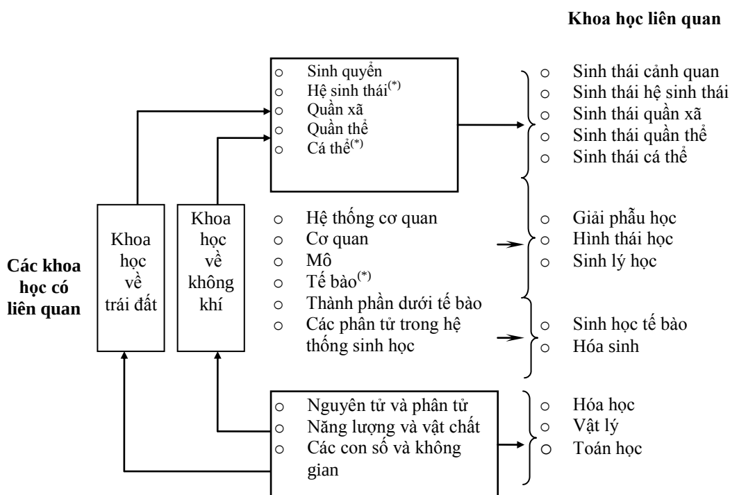
Hình 3.1. Các mức tổ chức sinh học và khoa học có liên quan (Rowe, 1961; Dẫn theo Kimmins, 1998).
