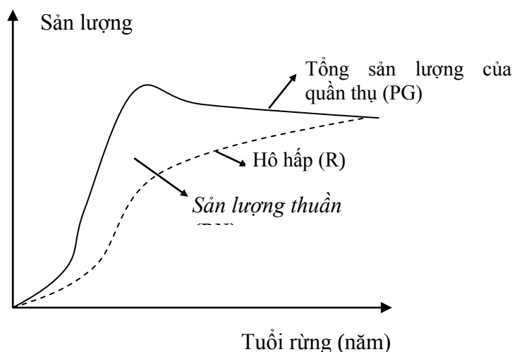
Hình 4.4. Sự biến đổi tổng sản lượng (PG), sản lượng thuần (PN) và sản lượng chi phí cho hô hấp (R) theo tuổi của rừng.
