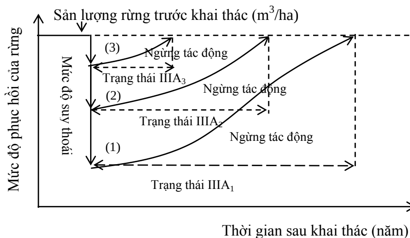
Hình 10.3. Sơ đồ mô tả rừng phục hồi lại sau khai thác chọn thô với cường độ khai thác khác nhau. Mũi tên hướng từ trục tung xuống dưới chỉ diễn thế thoái biến do ảnh hưởng của khai thác chọn. Mũi tên hướng từ trục hoành lên trên chỉ diễn thế phục hồi sau khai thác chọn.
