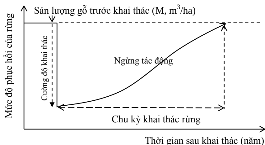
Hình 11.1. Sơ đồ mô tả chu kỳ khai thác rừng.
