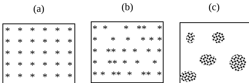
Hình 7.2. Những kiểu phân bố của các loài cây gỗ trên mặt đất.
