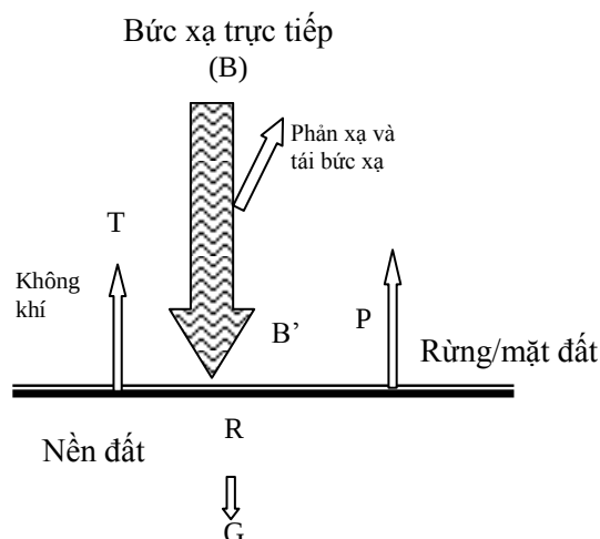
Hình 6.1. Sơ đồ cân bằng bức xạ ở rừng.
