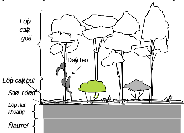
Hình 3.5. Những thành phần của rừng.
