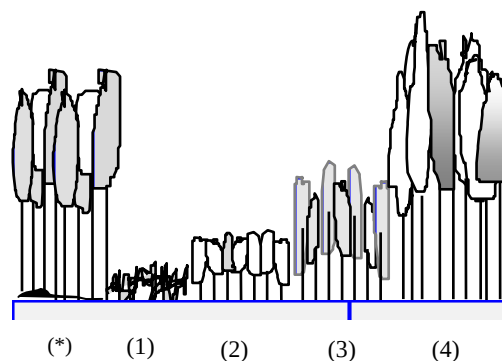
Hình 9.1. Sơ đồ biểu diễn một chuỗi diễn thế của rừng thứ sinh.
