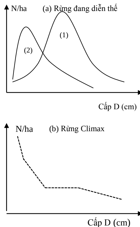
Hình 9.3. Phân bố N/D.
