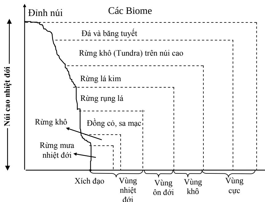
Hình 6.2. Các kiểu thảm thực vật phân bố theo độ cao và độ vĩ phân ánh các biên độ nhiệt độ và độ ẩm của không khí.
