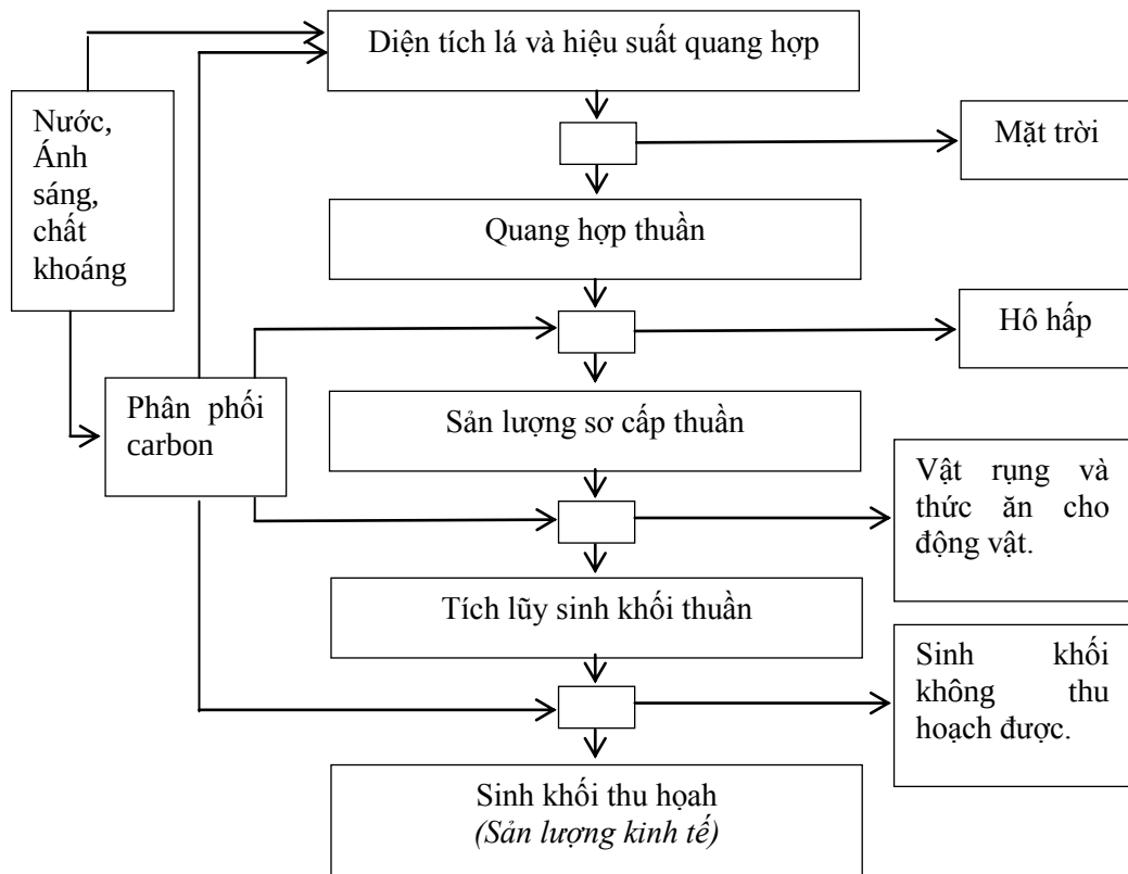
Hình 4.3. Những nhân tố ấn định sản lượng kinh tế của hệ sinh thái rừng ở một vùng khí hậu nhất định.
