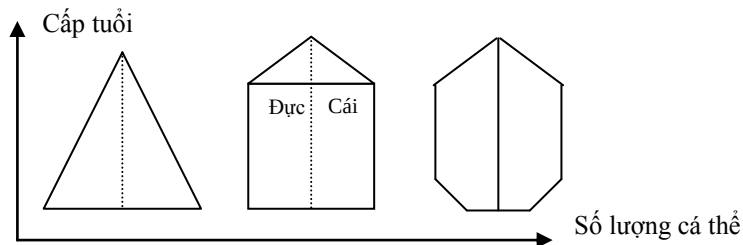
Hình 7.1. Các dạng tháp tuổi của quần thể: (a) phát triển; (b) ổn định; (c) giảm.
